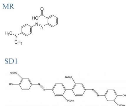
图3 两种取向材料MR和SD1的分子结构
