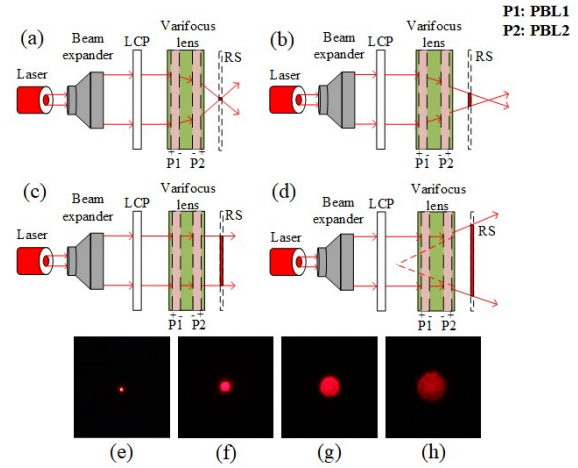
图13 (a)、(b)、(c)、(d)变焦透镜分别实现50、100、 \infty 、-100 cm焦距;(e)~(h)在接收屏上的图像 [43]
