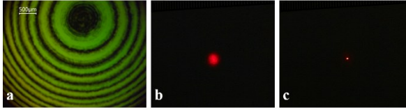
图 8 (a) PB 透镜的显微镜图;(b)(c)零电压和施加电压情况下 PB 透镜在 1 m 处的衍射图案
