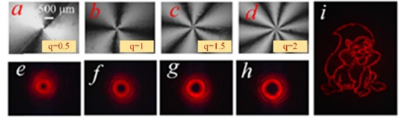
图 9(a)~(d) q=0.5, 1, 1.5, 2 的 q-plate 在偏光显微镜下的图像,及(e)~(h)对应生成的涡旋光束;(i)重建的 PB 全息图 [25]
