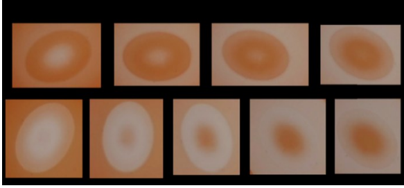
图5 在线偏振白光照明下旋转液晶盒观察到的不同图像 [25]
