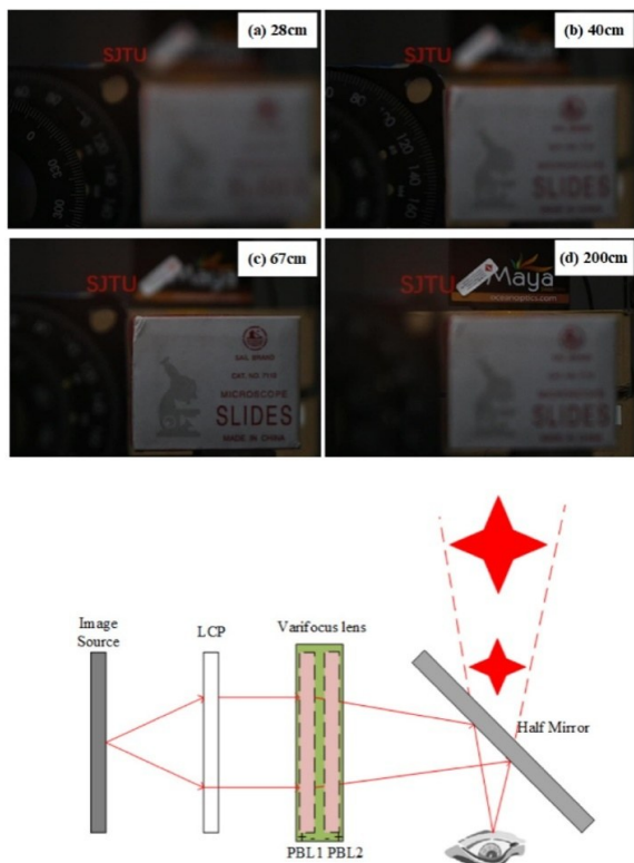
图14 “SJTU”分别成像在(a) 28 cm、(b) 40 cm、(c) 67 cm、(d) 200 cm的位置;(e) AR显示系统图 [43]
