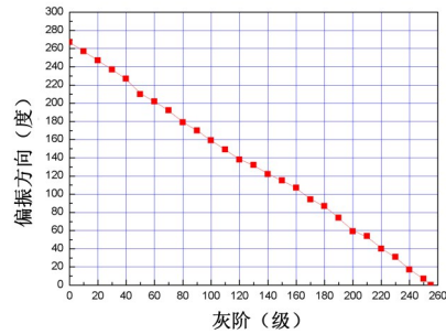
图 2 不同灰阶下的输出光偏振方向
